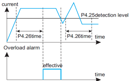
Рис.6-29 Сигнал о перегрузке
