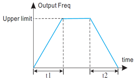
Рис.6-6 Время разгона/замедления
