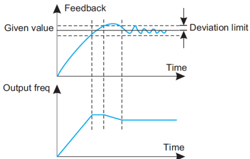
Рис.6-33 Предел отклонения
