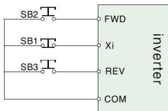
Рис.6-23 2-проводной режим управления 1
