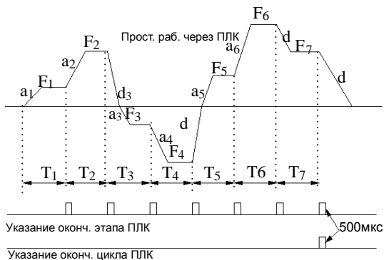
Рис.6-39 Простая работа через ПЛК
